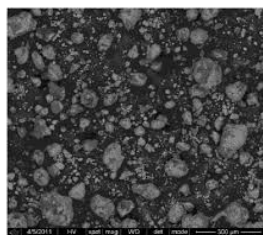
Fig 1. (d) SEM images of \text{TiO}_2 nanoparticles.
